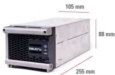
MÓDULO POTENCIA
