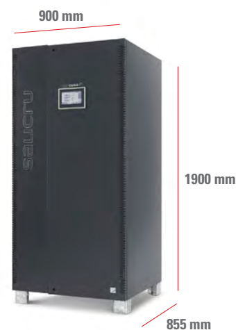
SLC-160/200-CUBE3+
